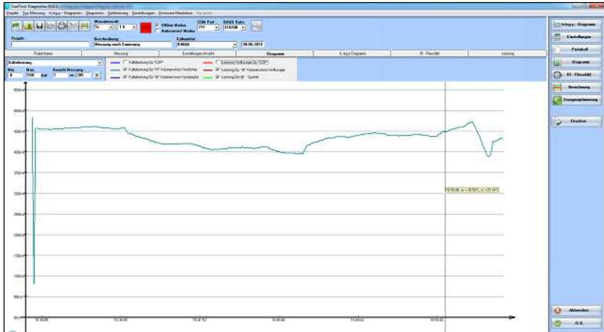
Abb. 10: Die gemessene Kälteleistung für das Gesamtsystem liegt nach dem Umbau im Mittel bei 429,8 kW.
